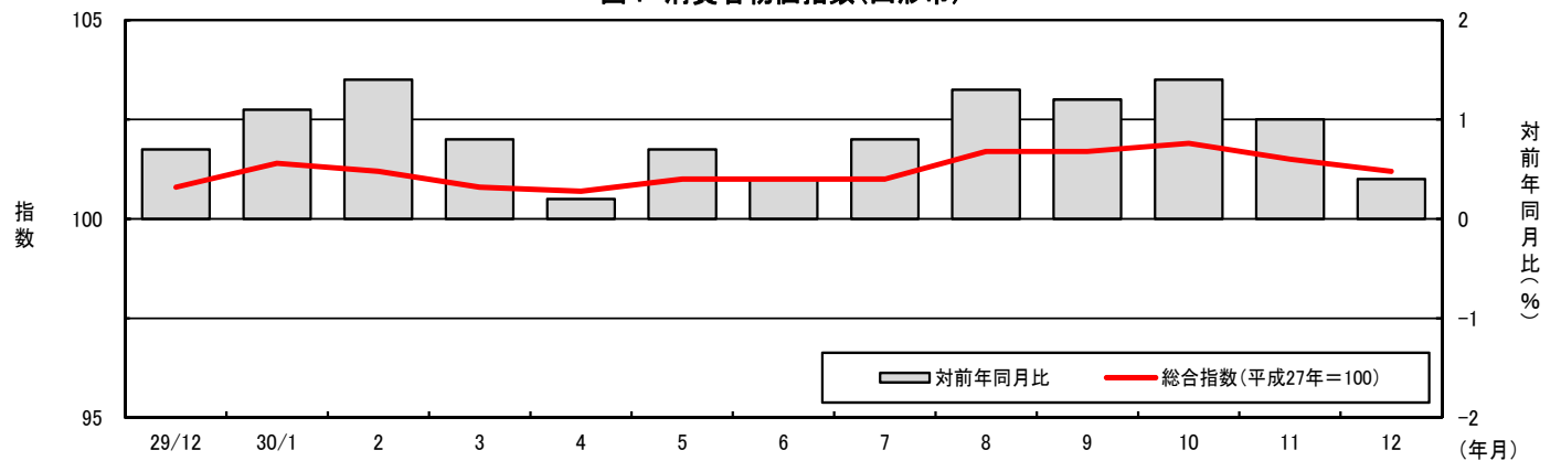
図4 消費者物価指数(山形市)
